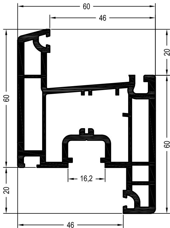
Профили створок
